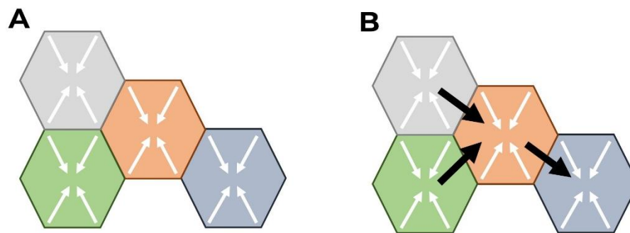
Fig. 4. Modelos conceptuales de los Ordenamientos Ecológicos Territoriales (OET) y los PAMIC. A) Modelo conceptual de la caracterización y análisis de las unidades de planeación de los OET considerando únicamente sus atributos internos (flechas blancas). B) Modelo conceptual de los PAMIC con base en el análisis de la vinculación e interconexión entre las unidades de planeación asociada a la red de flujo superficial de las cuencas (flechas negras).
