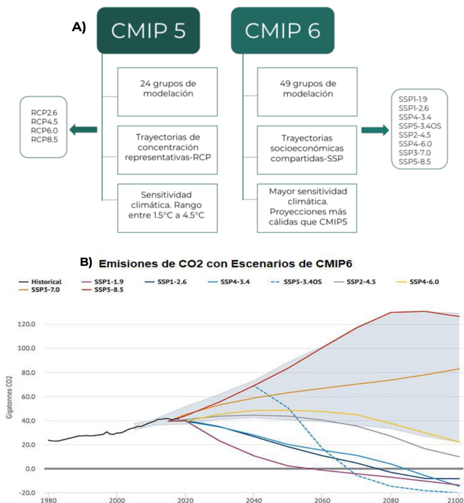
Fig. 15. Principales diferencias entre CMIP5 y CMIP6 (INECC, 2022). B) Escenarios futuros de emisiones de CO 2 descritos en CMIP6, incluyendo emisiones históricas de CO 2 (en color oscuro). El área sombreada representa el intervalo de escenarios de referencia sin políticas (Hausfather, 2019).
