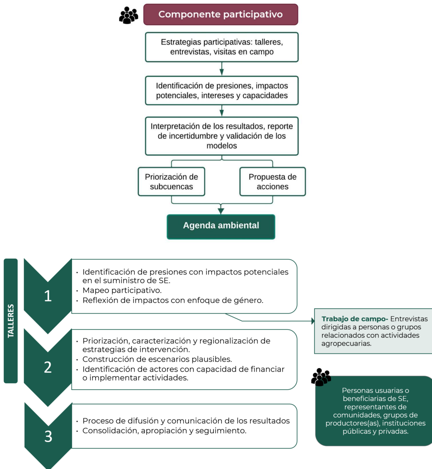
Fig. 7. Esquema conceptual del componente participativo de los PAMIC.
