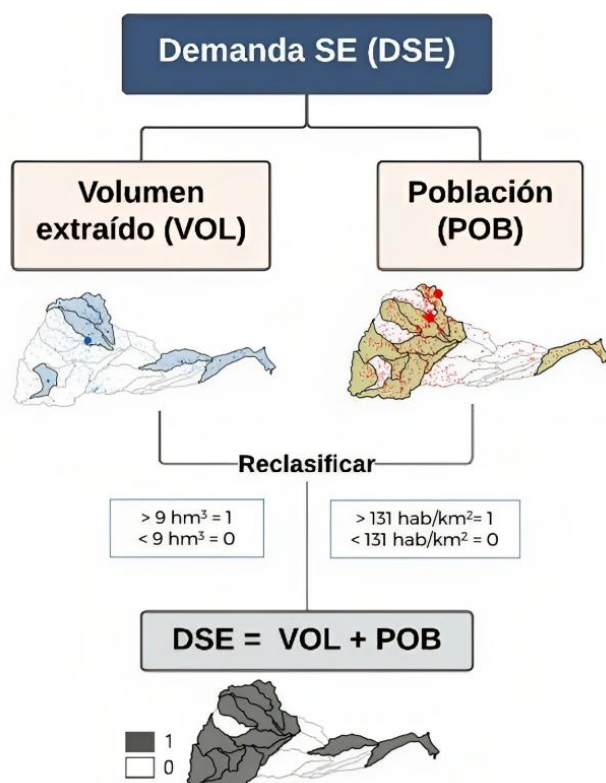
Fig. 13. Esquema de integración y análisis para la identificación de las subcuencas (resaltadas en color oscuro) con mayores volúmenes de extracción de agua y densidad poblacional.
