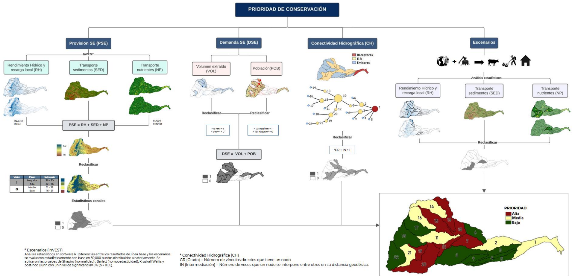
Fig. 21. Ejemplo del esquema de integración y análisis para la priorización territorial: identificación de subcuencas prioritarias para la implementación de acciones de conservación en la cuenca del RLA.
