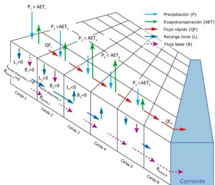
Fig. 11. Esquema conceptual para el cálculo del balance hídrico a escala de píxel, utilizado en el modelo de rendimiento hídrico estacional (InVEST) (Hamel et al., 2020).
