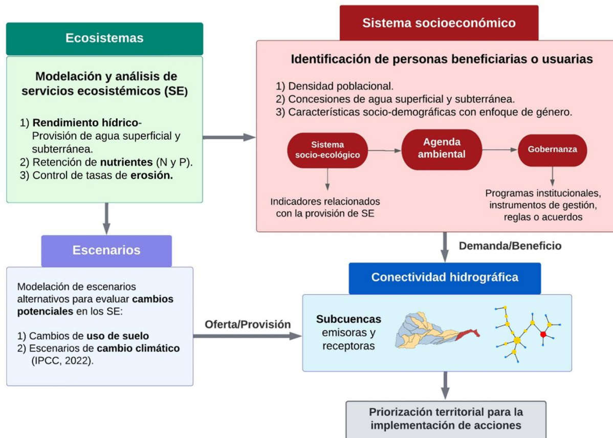
Fig. 6. Esquema conceptual del componente técnico de los PAMIC.
