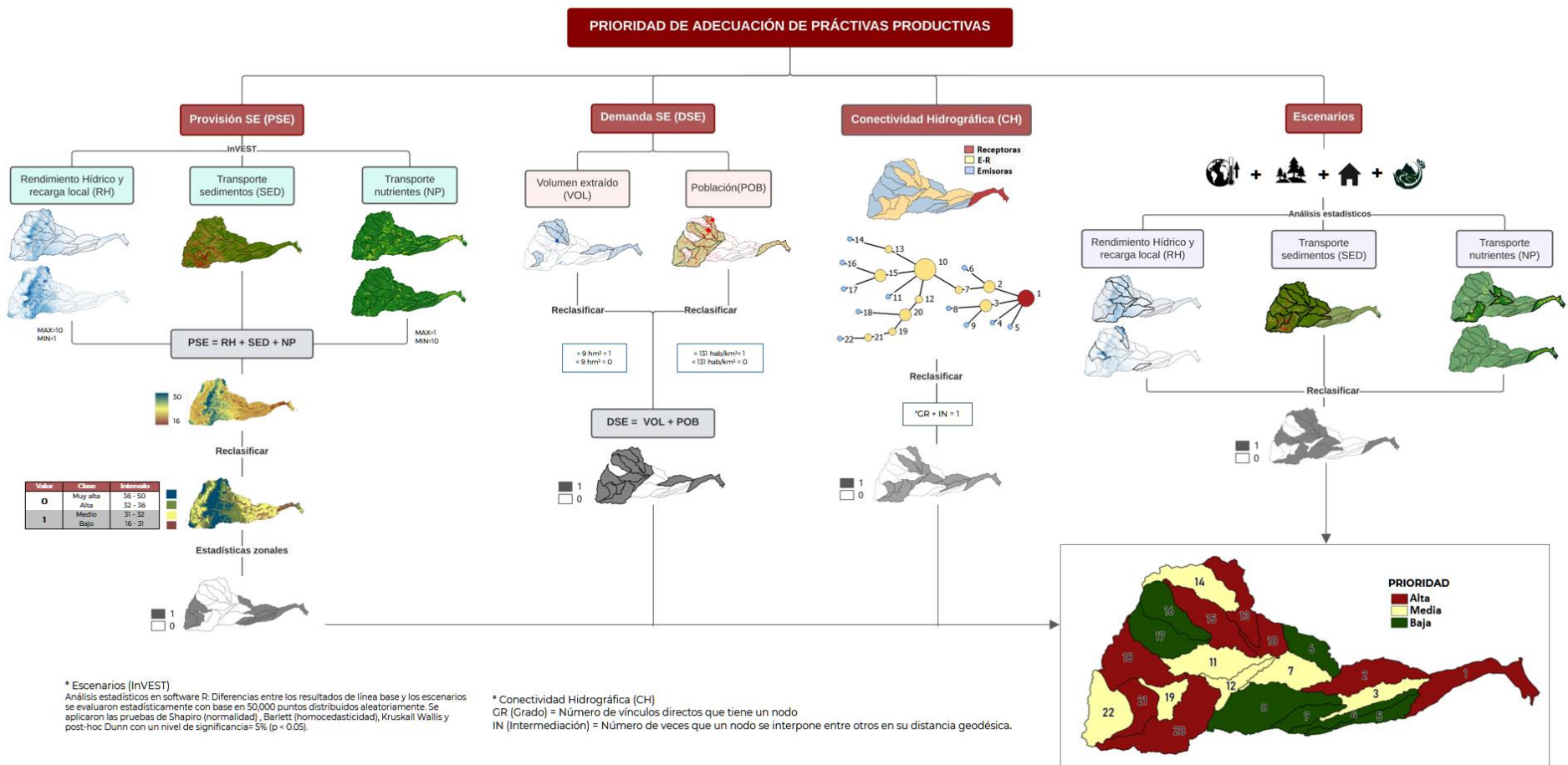
Fig. 23. Ejemplo del esquema de integración y análisis para la priorización territorial: identificación de subcuencas prioritarias para la implementación de acciones de restauración o rehabilitación en la cuenca del R
